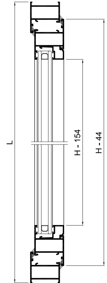
Sección B-B'
