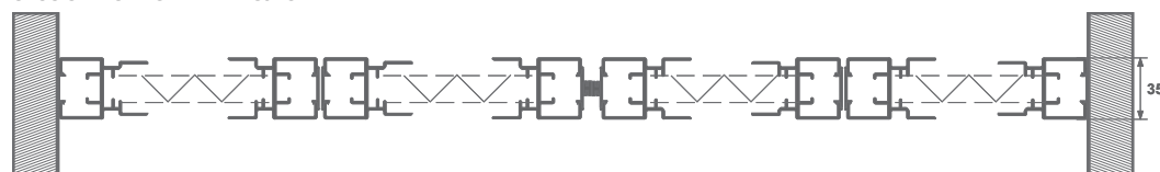
SECCIÓN HORIZONTAL 4 HOJAS
