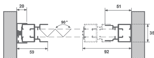
SECCIÓN HORIZONTAL 2 HOJAS
