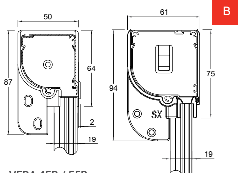
VERA 45B / 55B Cubrecabezal monobloque para una instalación práctica y veloz.
