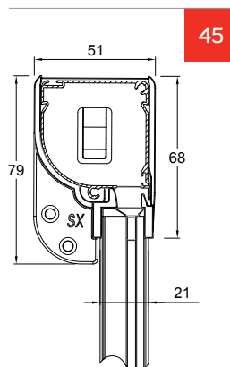
Versión con guías telescópicas laterales que facilitan un deslizamiento perfecto incluso en huecos que no cuadran perfectamente.
