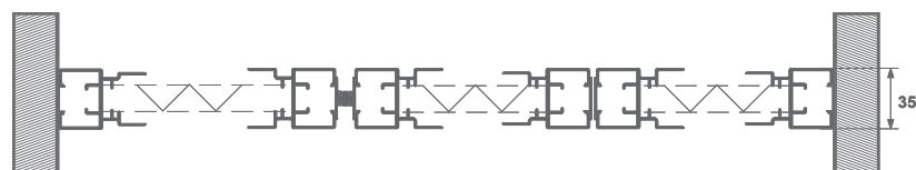
SECCIÓN HORIZONTAL 3 HOJAS
