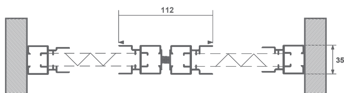
SECCIÓN HORIZONTAL 1 HOJA
